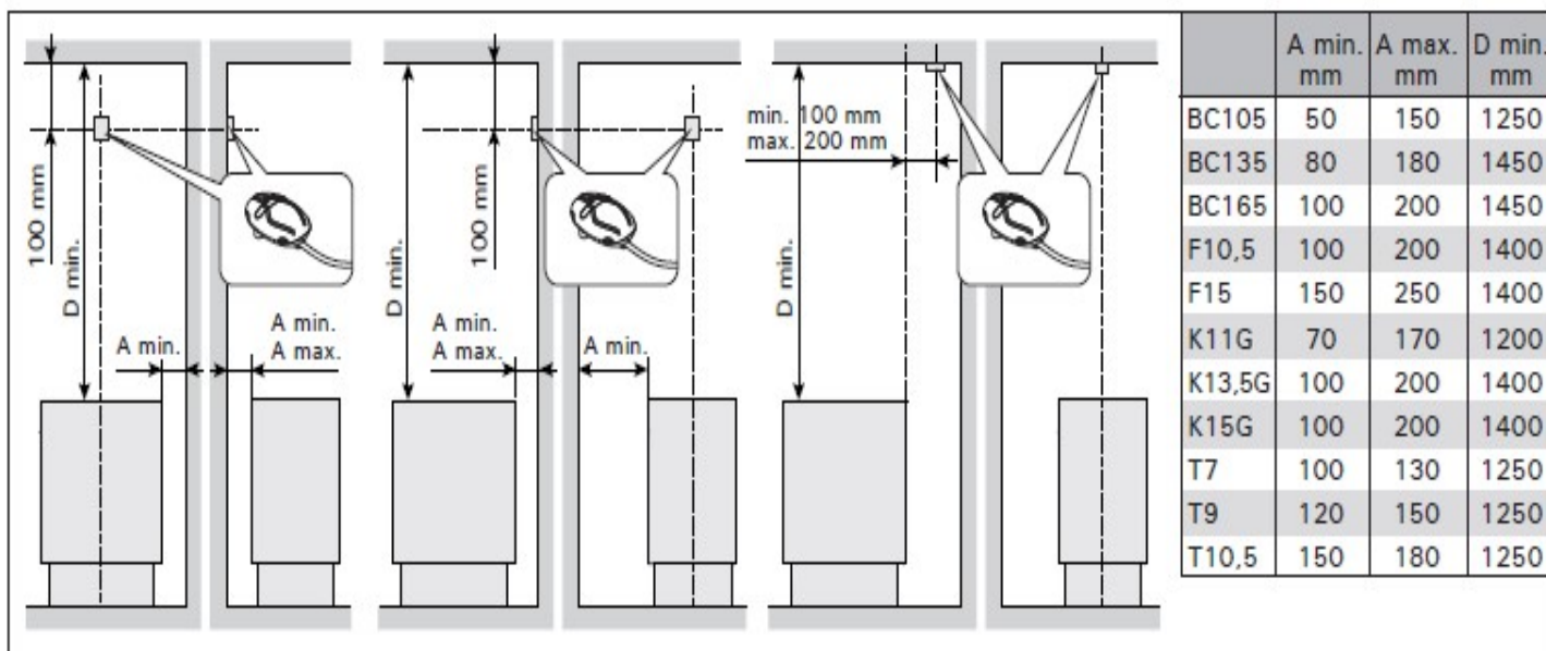
obr. 5: Umístění senzoru při použití kamen postavených na podlaze sauny.
