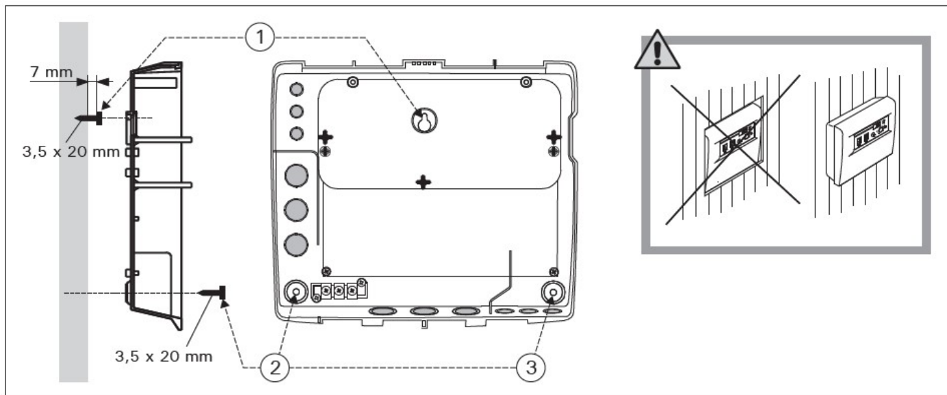
obr. 2: Instalace řídící jednotky na stěnu Figure 2: Wall-mounting the control unit
