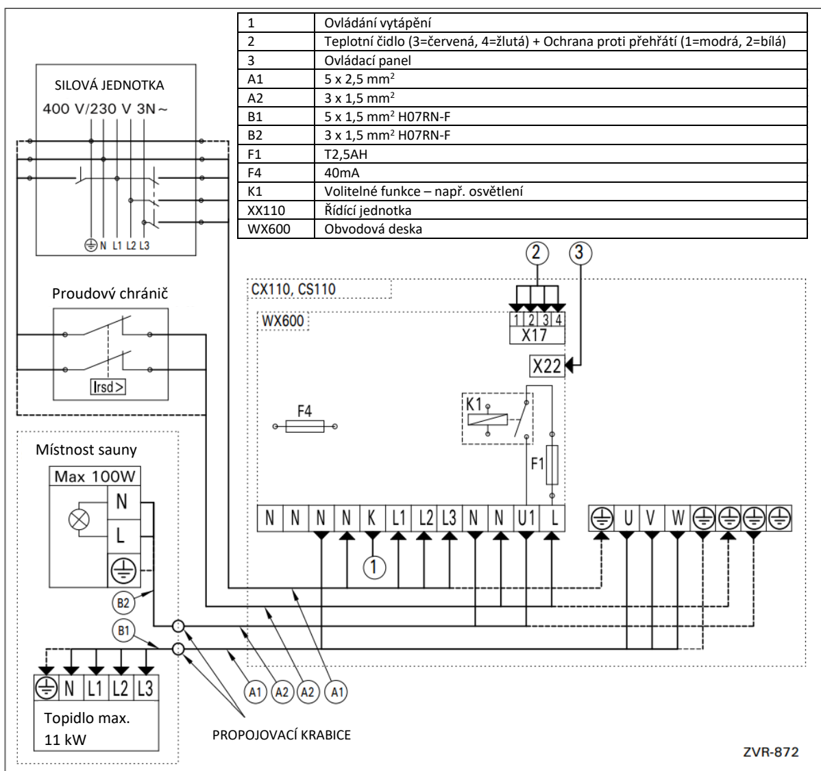
Obrázek 6. Elektrické zapojení
